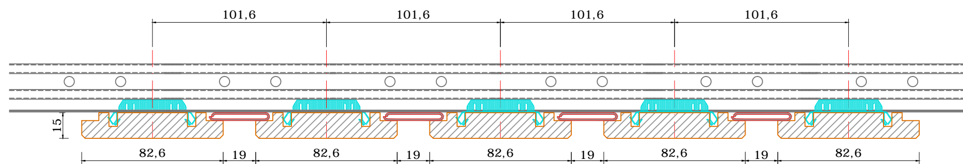
Doorsnede B-B
